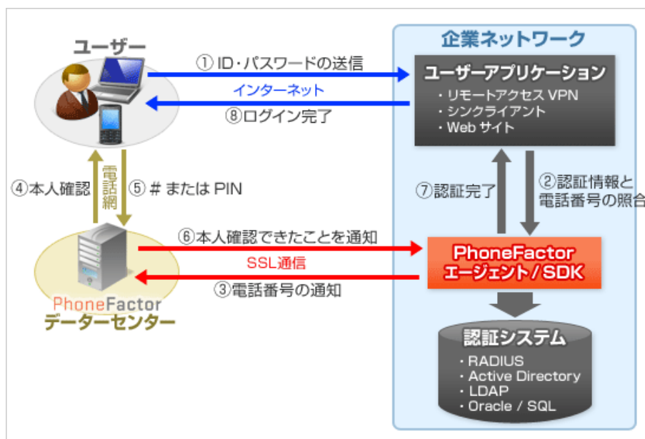
図1: PhoneFactor の認証のしくみ
