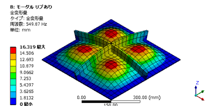
リブを立て面の振動を抑える
