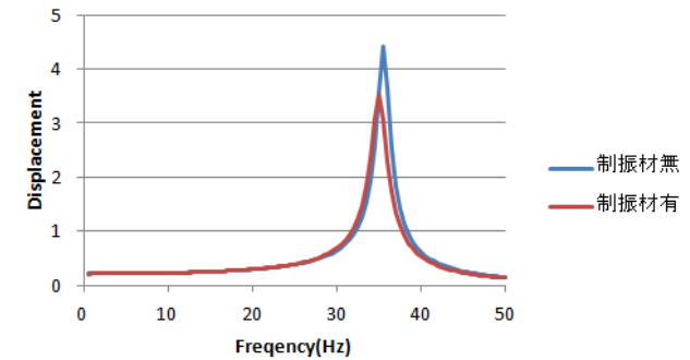
平板中心部の変位応答図
